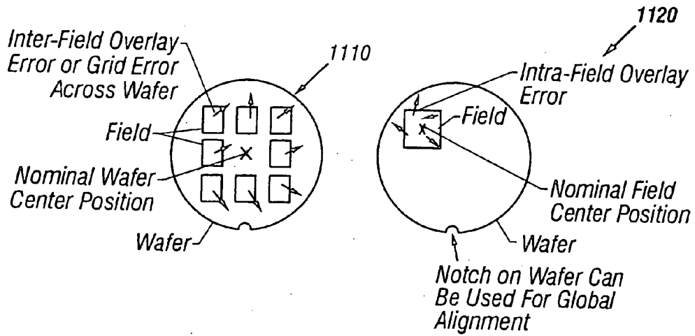
FIG. 11A
