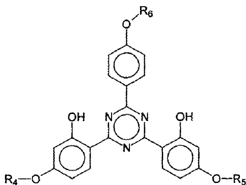
(BIS-RESOR-TRIAZIN)-I
