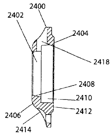
A-A FIG. 11c
