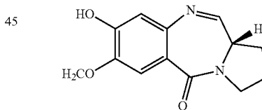
DC-81
