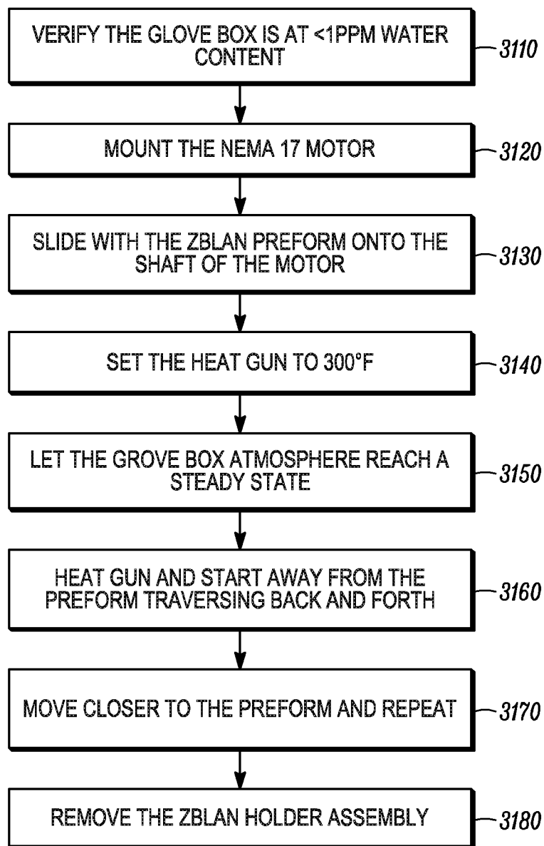
FIG. 31
