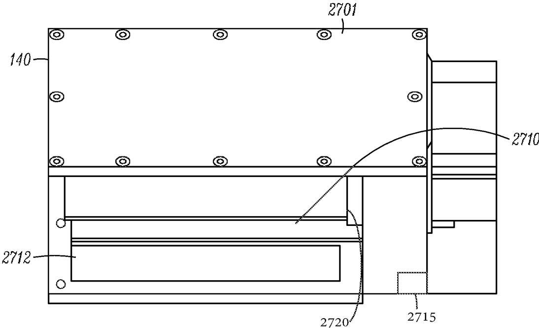
FIG. 26A
