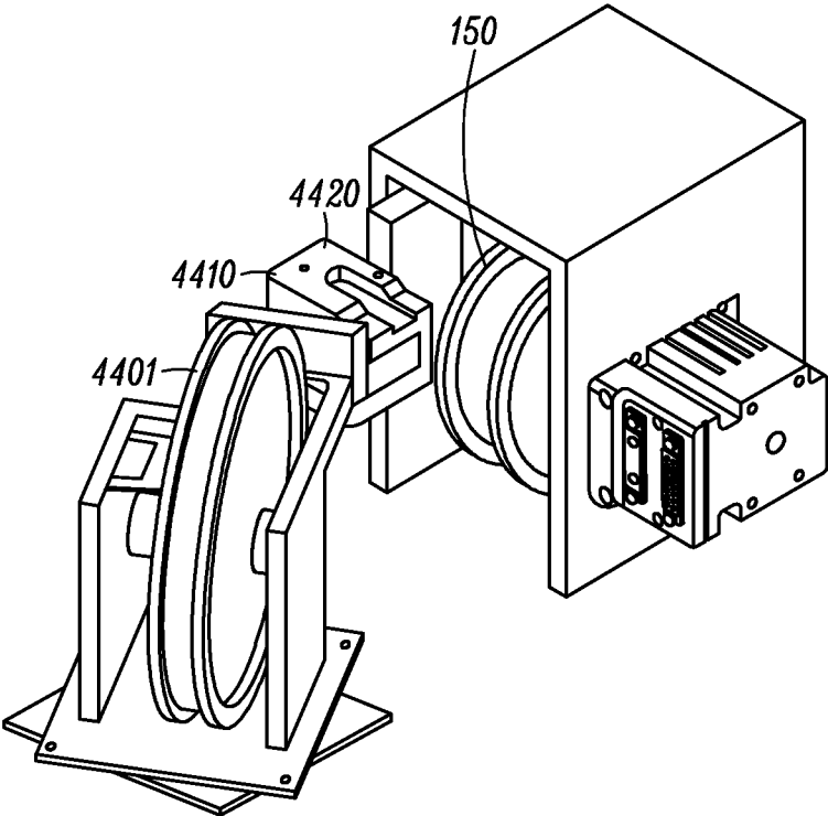
FIG. 44
