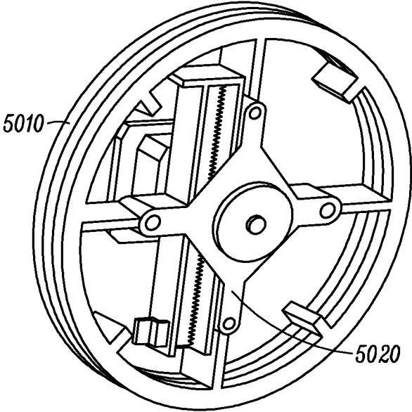
FIG. 50A
