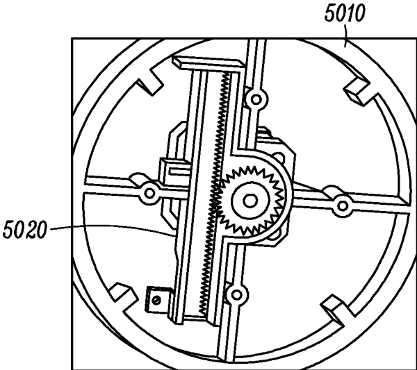
FIG. 50B
