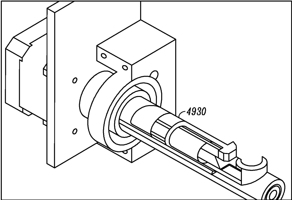
FIG. 49A
