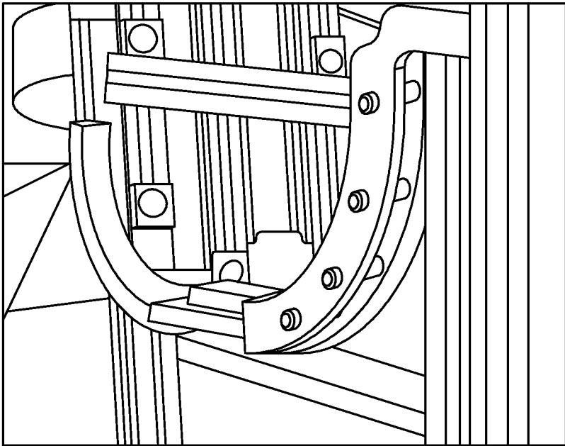
FIG. 42B
