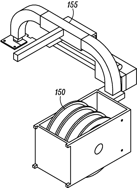
FIG. 45B
