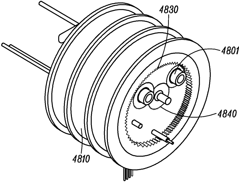
FIG. 48C
