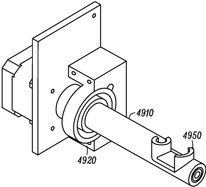
FIG. 49B
