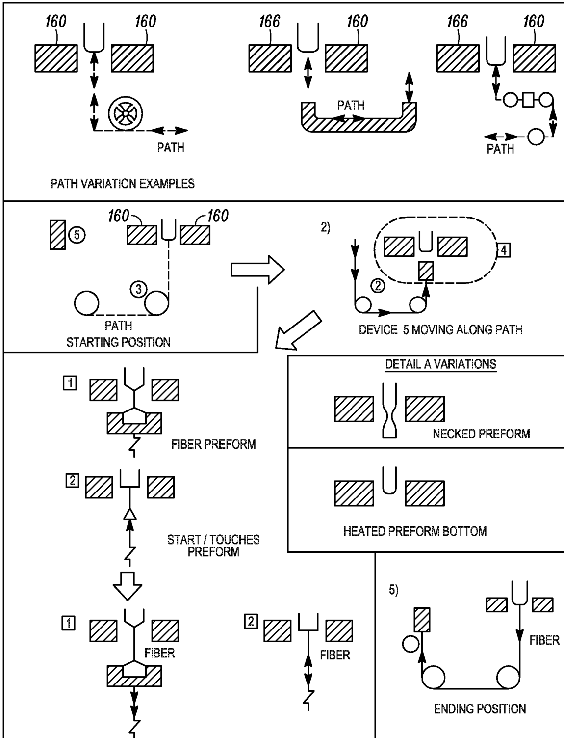
FIG. 53
