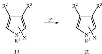
Scheme VI
