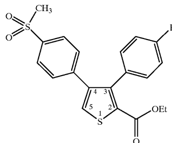
Ethyl[4-(4-methylsulfonylphenyl)-3-(4-fluorophenyl)thien-2-yl]carboxylate
