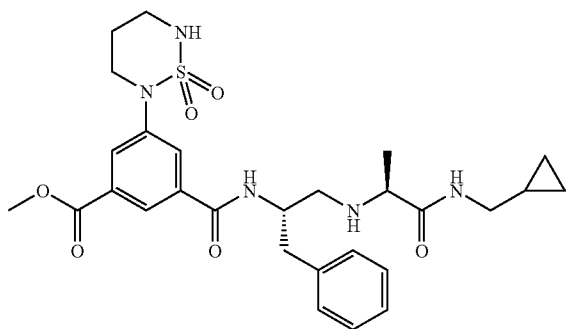
1-j
