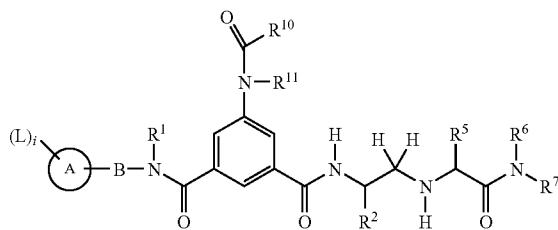
(Id)
