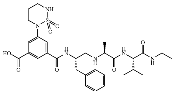
1-k
