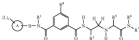
(Ib)
