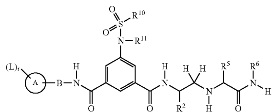
(Ie)
