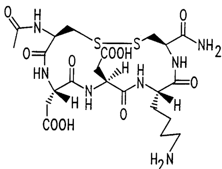
N-Ac-CDDKC-NH 2
