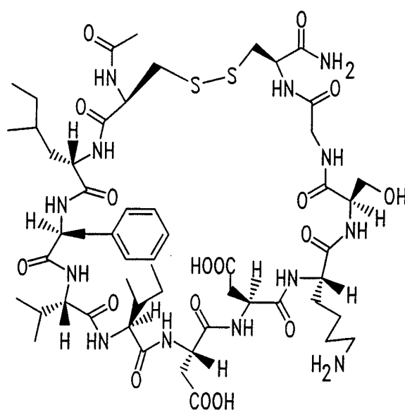
N-Ac-CIFVIDDKSGC-NH 2
