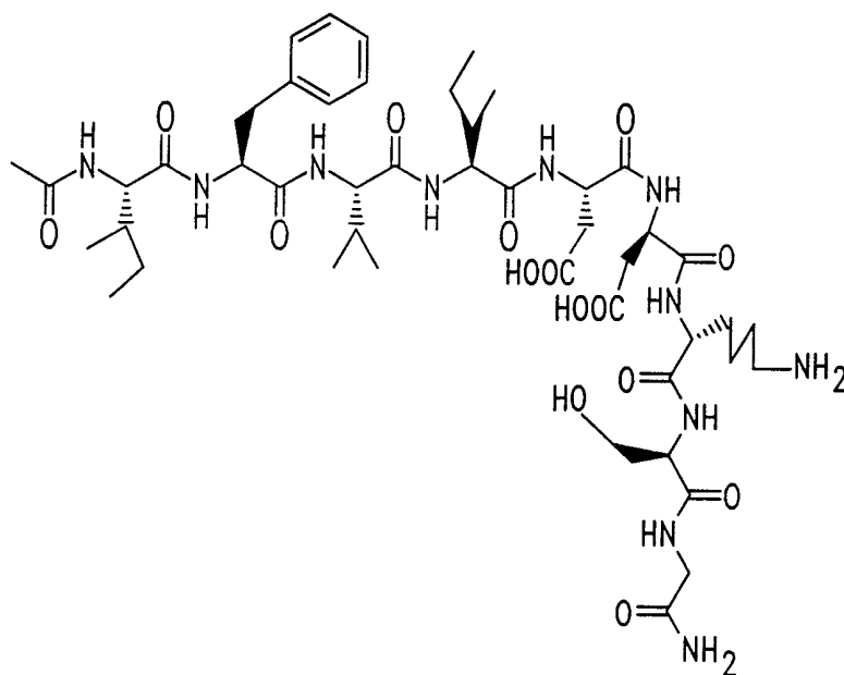
N-Ac-IFVIDDKSG-NH 2
