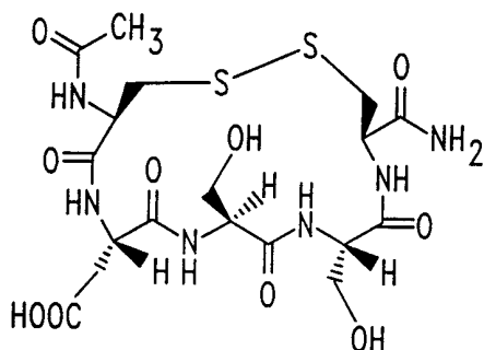
N-Ac-CDSSC-NH 2
