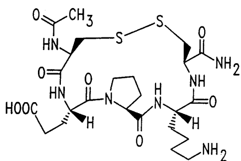
N-Ac-CEPKC-NH 2
