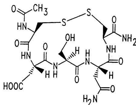
N-Ac-CDSNC-NH 2
