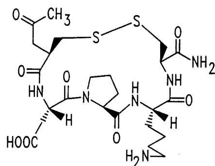
N-Ac-CDPKC-NH 2
