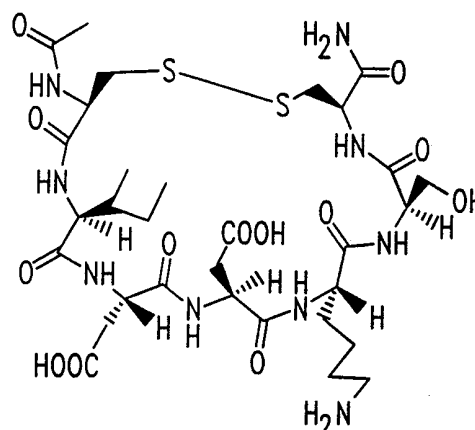
N-Ac-CIDDKSC-NH 2
