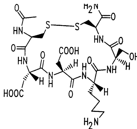
N-Ac-CDDKSC-NH 2
