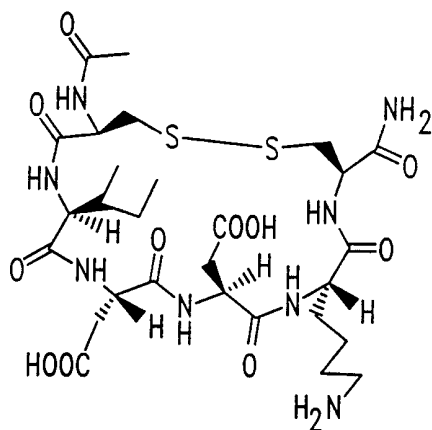
N-Ac-CIDDKC-NH 2
