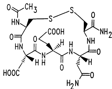
N-Ac-CDENC-NH 2
