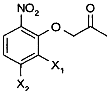
allgemeine Formel 1
