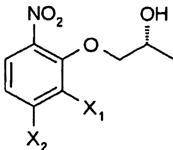
allgemeine Formel 2
