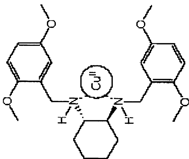
(S,S)-1-Cu II
