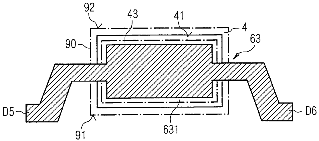
FIG 2 A-A
