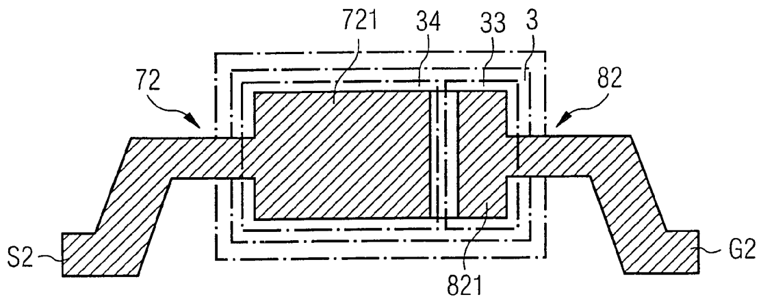
FIG 3 B-B
