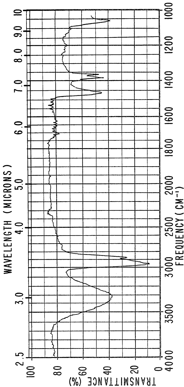
IR SPECTRUM FOR EXAMPLE II, DIISOUNDECANOL.
