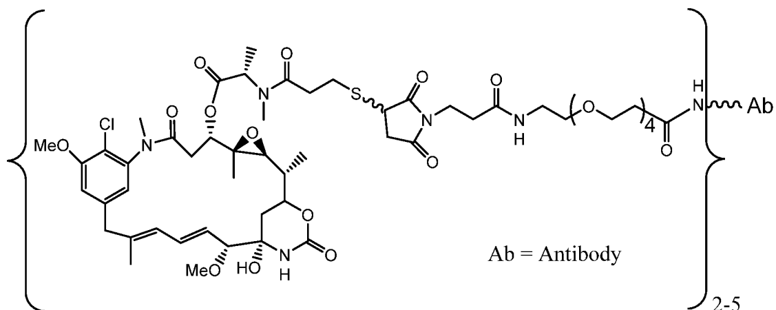
Ab-PEG4-Mal-DM1
