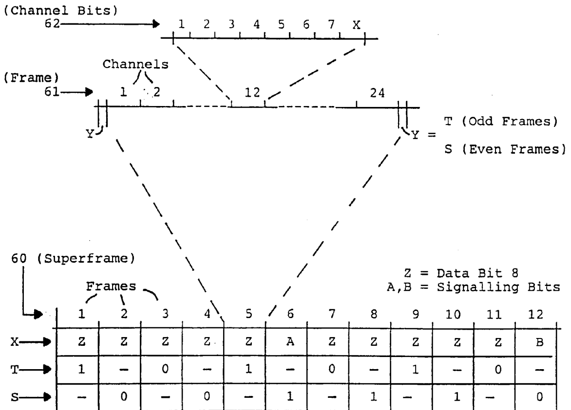
Fig. 7 (T-1 Frame Format)
