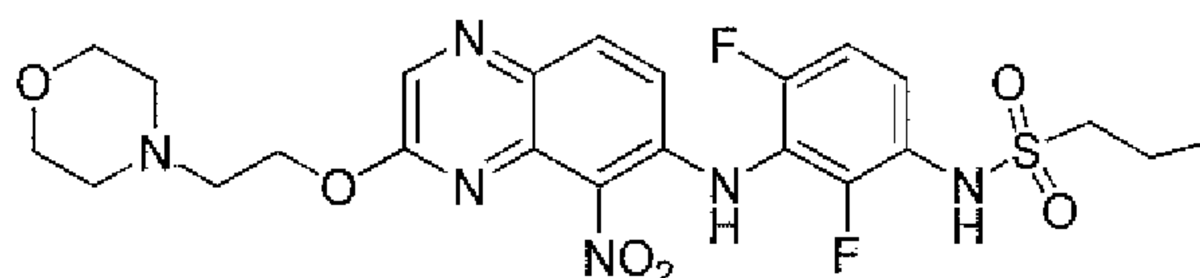
N1-(2,4-difluoro-3-[(3-(2-morpholinoethoxy)-5-nitro-6-quinoxaliny)amino]phenyl)-1-propanesulfonamide
