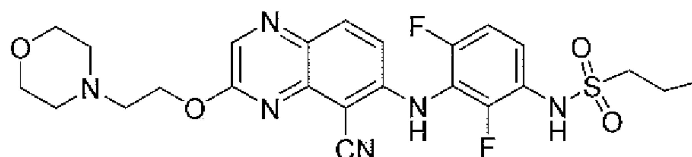
N1-(3-([5-cyano-3-(2-morpholinoethoxy)-6-quinolaliny]amino)-2,4-difluorophenyl)-1-propanesulfonamide
