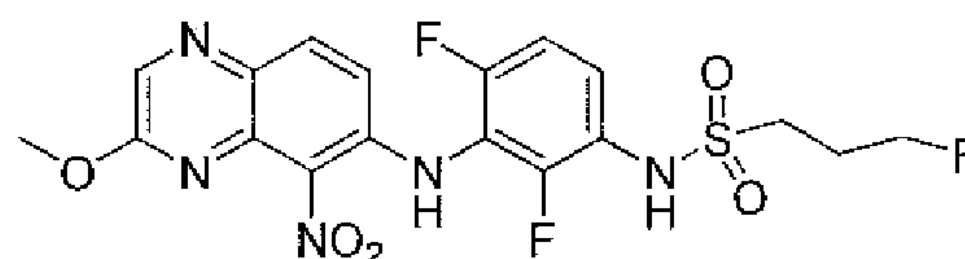
N1-(2,4-difluoro-3-[(3-methoxy-5-nitro-6-quinoxaliny)amino]phenyl)-3-fluoro-1-propanesulfonamide
