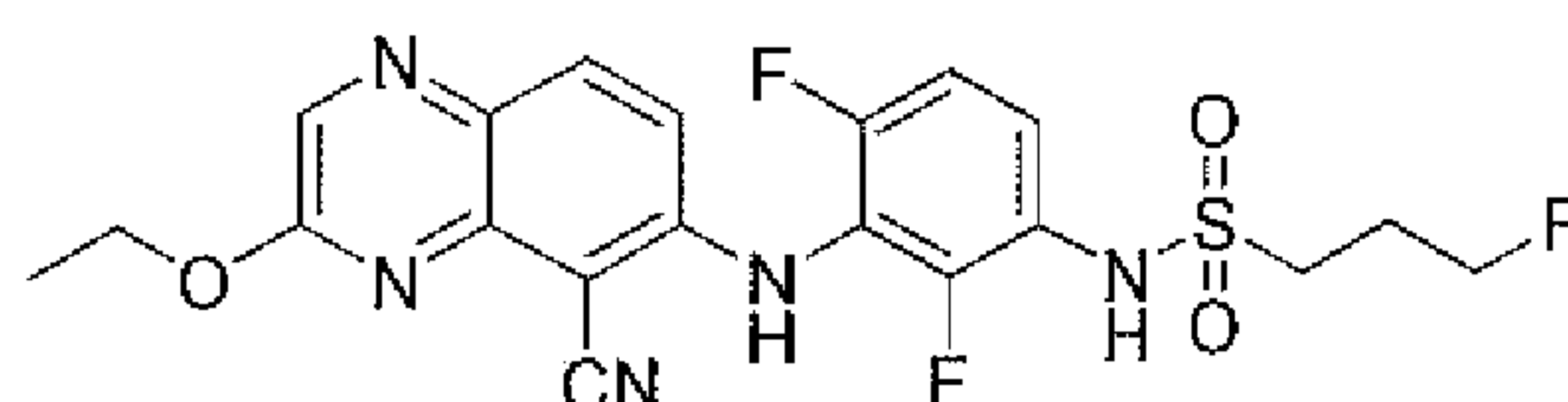
N -(3-(5-cyano-3-ethoxyquinoxalin-6-ylamino)-2,4-difluorophenyl)-3-fluoropropane-1-sulfonamide
