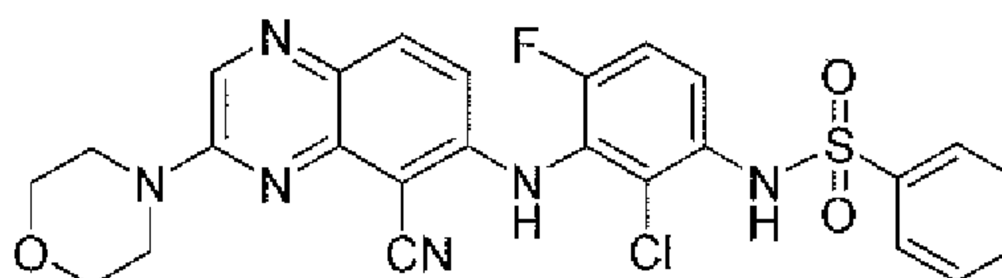
N -(2-chloro-3-(5-cyano-3-morpholinoquinoxalin-6-ylamino)-4-fluorophenyl)benzenesulfonamide
