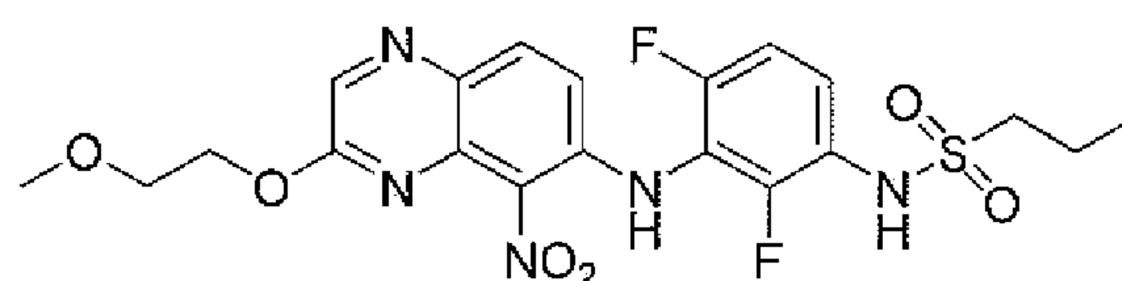
N1-(2,4-difluoro-3-[3-(2-methoxyethoxy)-5-nitro-6-quinoxaliny]aminophenyl)-1-propanesulfonamide
