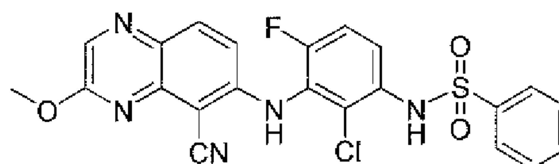
N -(2-chloro-3-(5-cyano-3-methoxyquinoxalin-6-ylamino)-4-fluorophenyl)benzenesulfonamide
