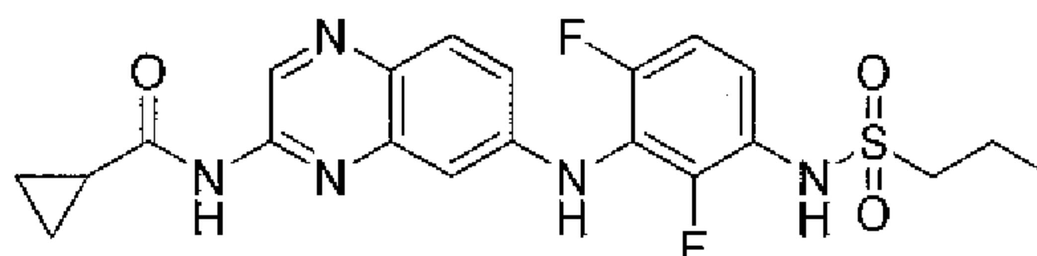
N1-(7-[2,6-difluoro-3-[(propylsulfonyl)amino]anilino]-2-quinoxaliny)-1-cyclopropanecarboxamide
