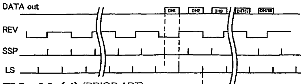
FIG. 26 (d) (PRIOR ART)
