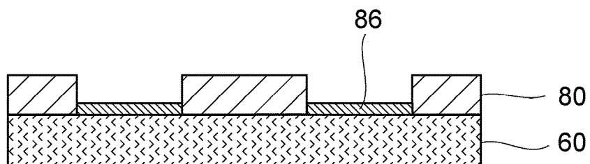
FIG.49
