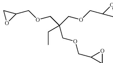
Denacol EX321L 2,2'-(((2-ethyl-2-((oxiran-2-ylmethoxy)methyl)propane-1,3-diyl)bis(oxy))bis(methylene))bis(oxirane)
