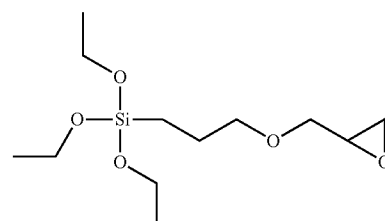
3-GTS (KBM-403E) triethoxy(3-(oxiran-2-ylmethoxy)propyl)silane
