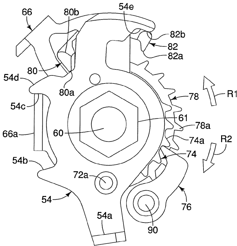
FIG. 29
