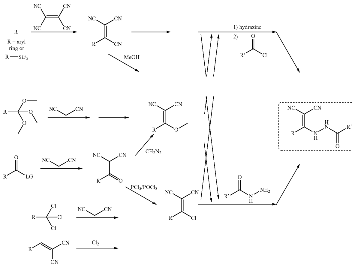
Scheme IV:
