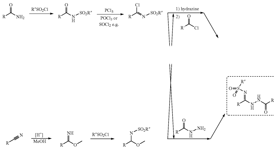
Scheme III:
