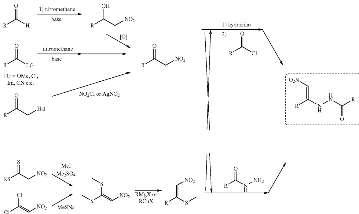
Scheme VI:
