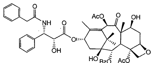
Taxol F
