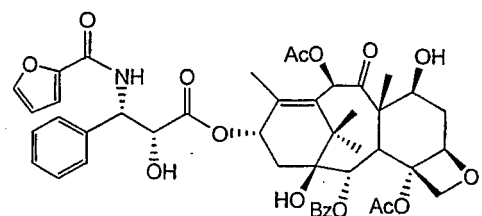
Taxol G
