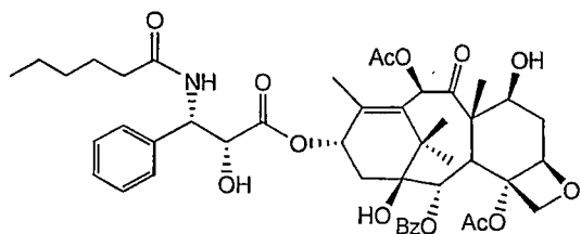
Taxol C
