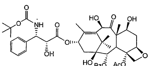
Docetaxel
