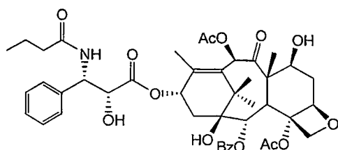
Taxol D
