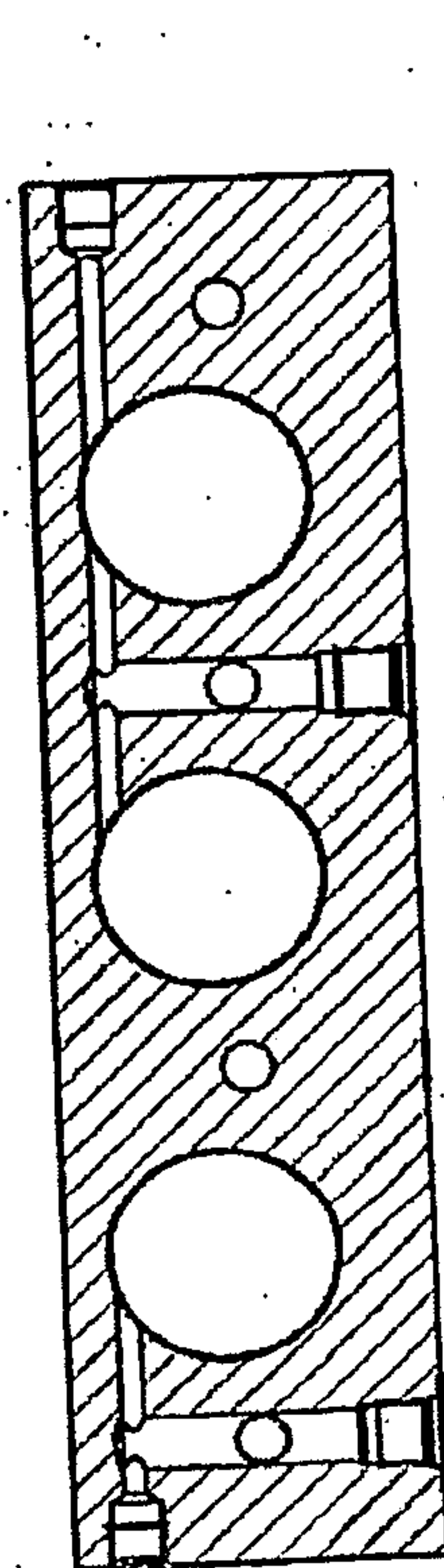
SECTION D-D FIG. 10D
