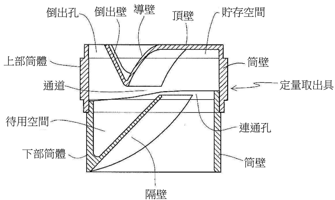
【放大剖面參考圖】
