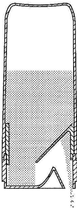
【使用狀態參考圖7】
