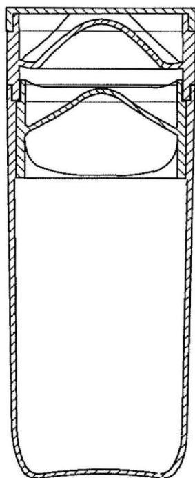
【A-A線剖面圖】
