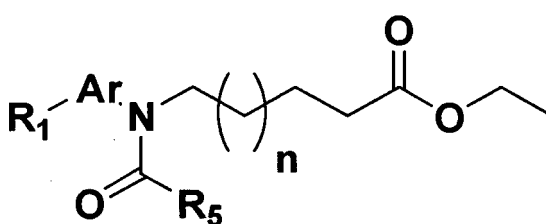
[Formula VIII]
