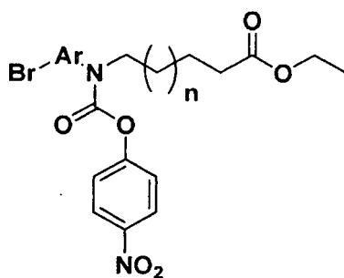
[Formule VI]
