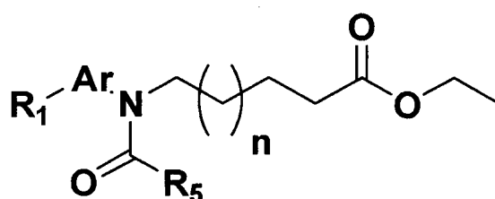
[Formula VIII]
