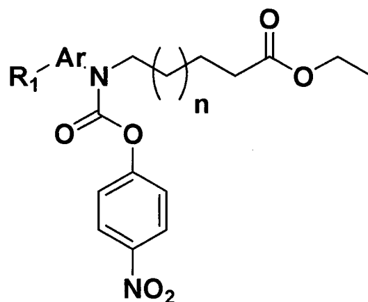
[Formula VII]
