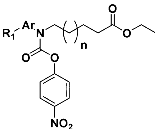
[Formula VIII]
