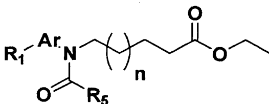
[Formule VIII]
