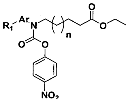
[Formule VII]
