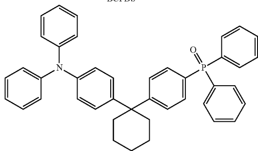
POPCPA
