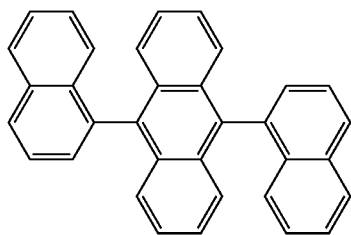
POPCPA
