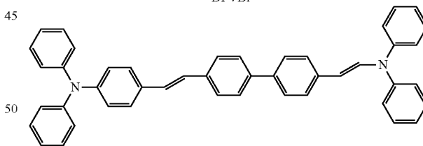
DPVBi
