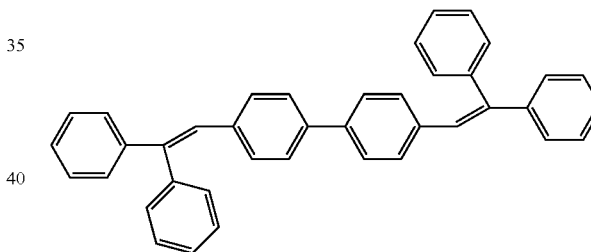
DPVBi
