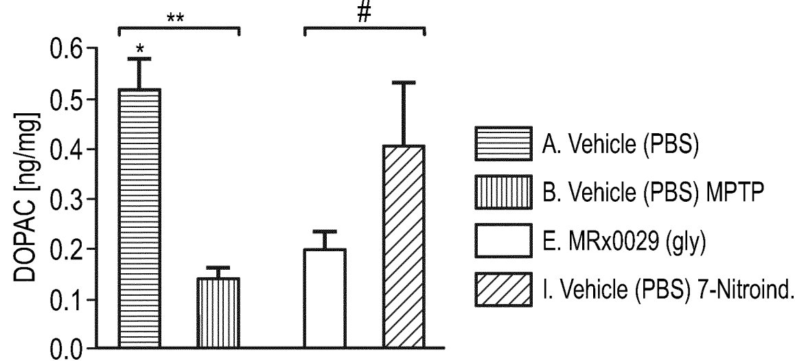
FIG. 12B DOPAC
