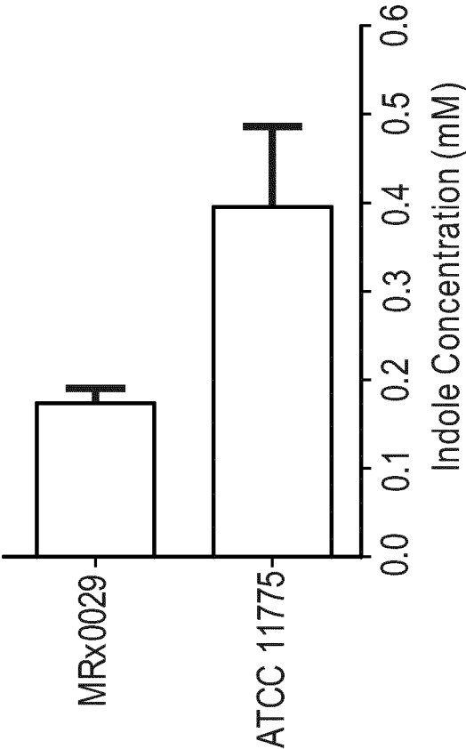
FIG. 10 Indole Assay
