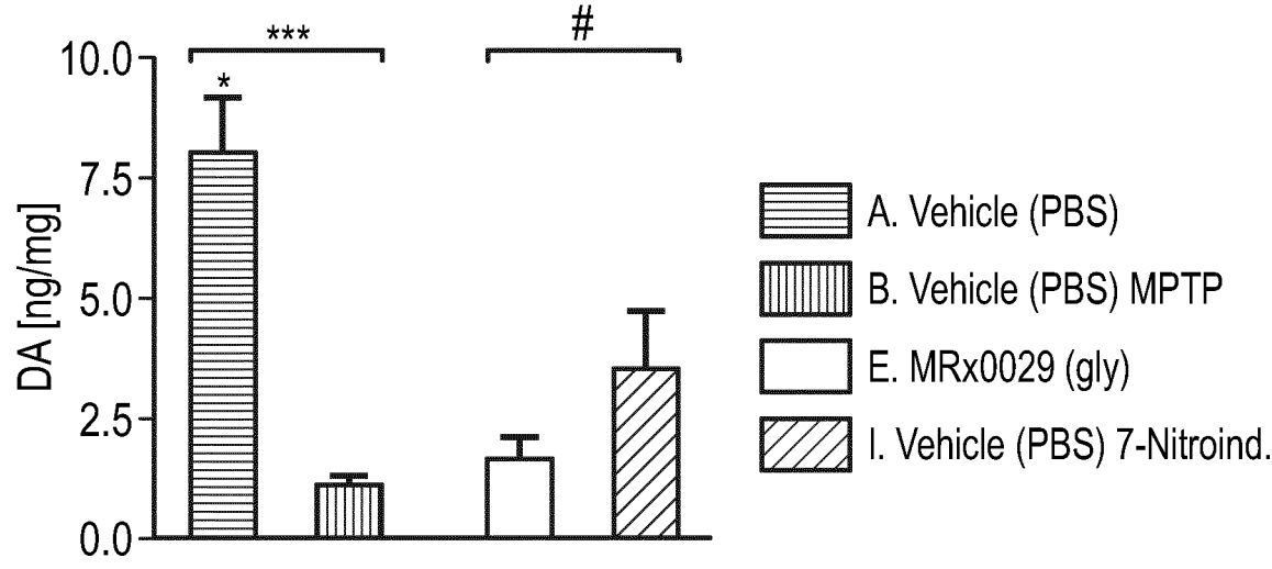
FIG. 12A DA
