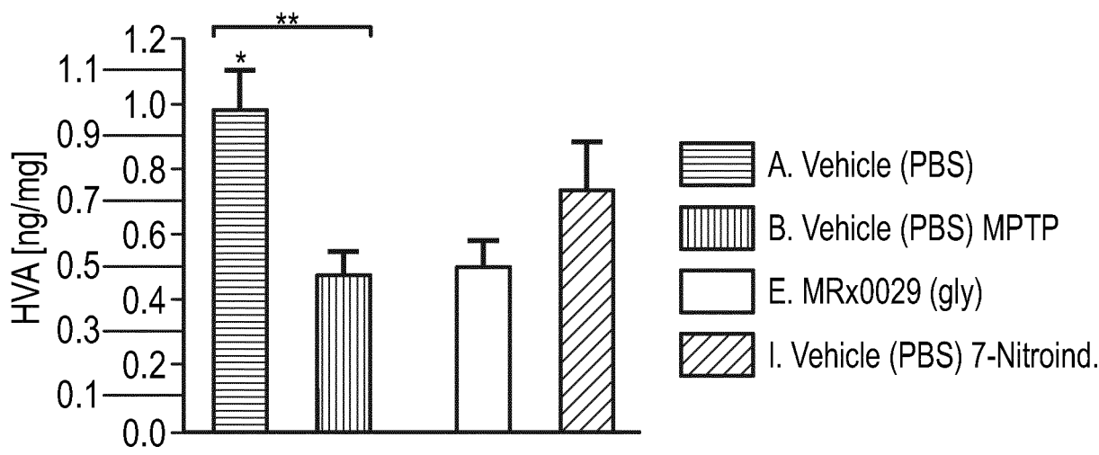
FIG. 12C HVA
