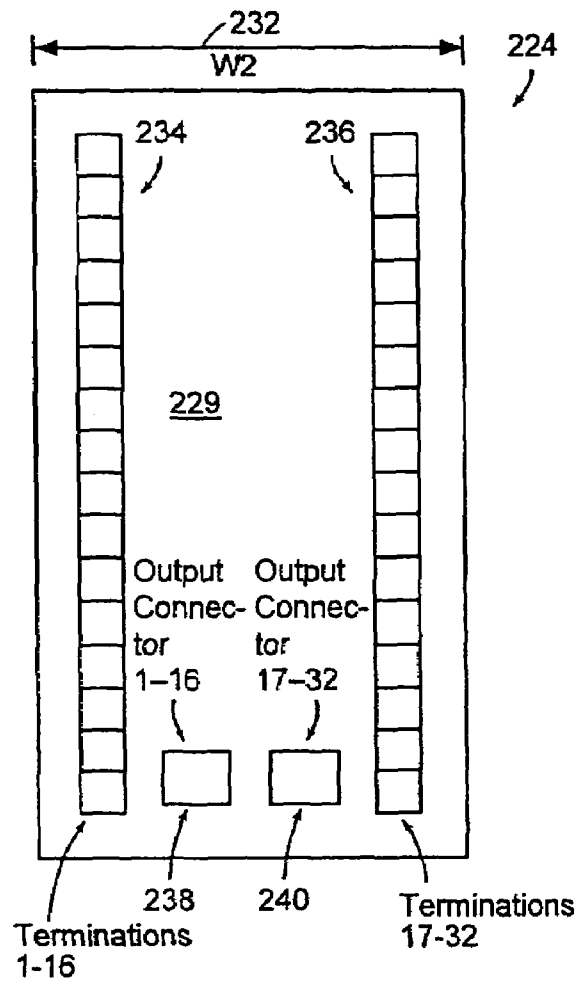
32 Output Module
