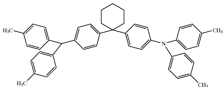
TPAC
