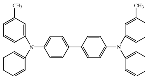
TPD
