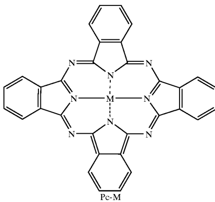
Pc-M
