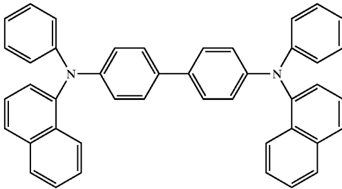
\alpha -NPD
