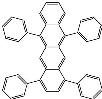
Rubrene
