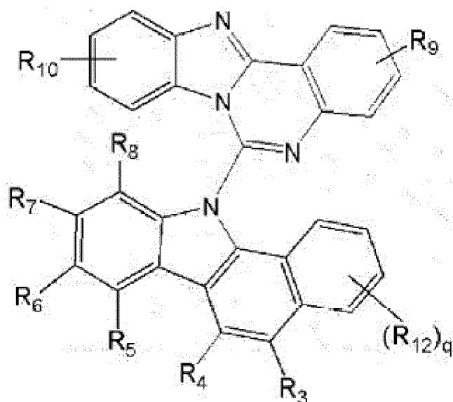
[Formule chimique 3]
