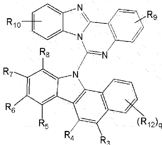
[chemische Formel 3]
