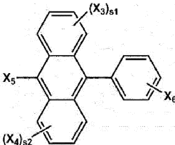
[Formule chimique 5]
