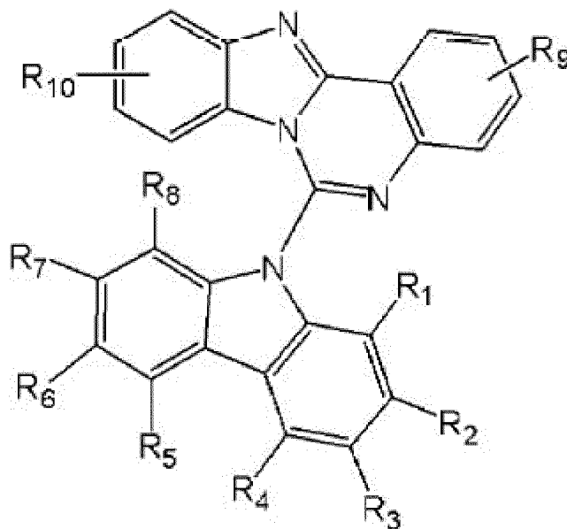
[Formule chimique 1]
