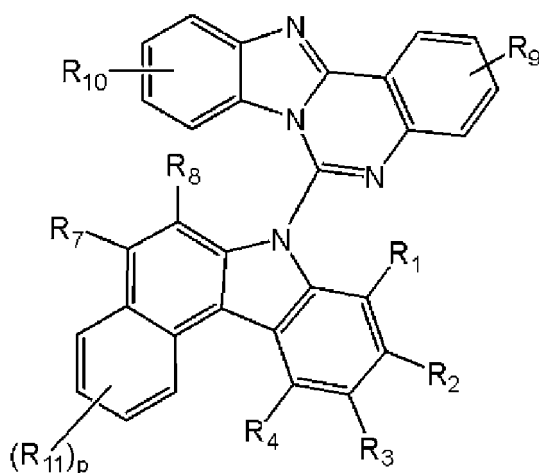
[chemische Formel 3]
