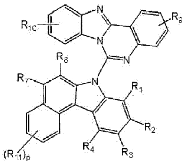
[Formule chimique 2]
