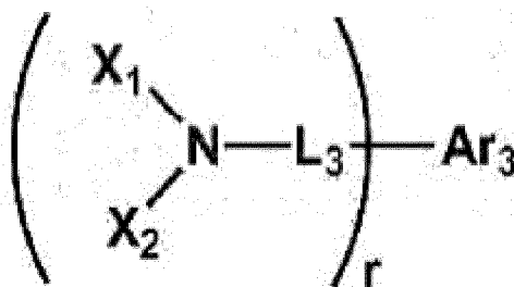
[Formule chimique 4]
