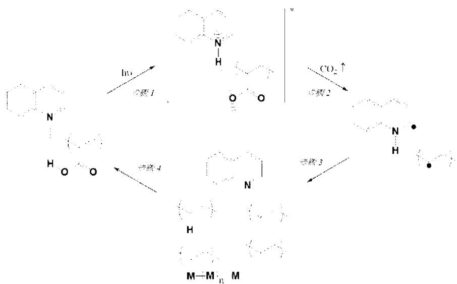
【0253】 [化學式 7]
