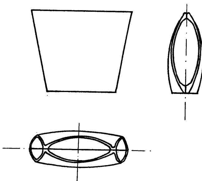
rys.2 rzuty spinki
