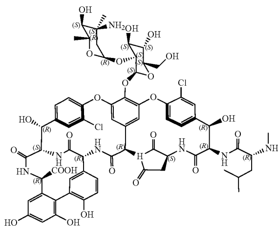
DAmS (Des-(amido)-succinimido-Vancomycin B)
