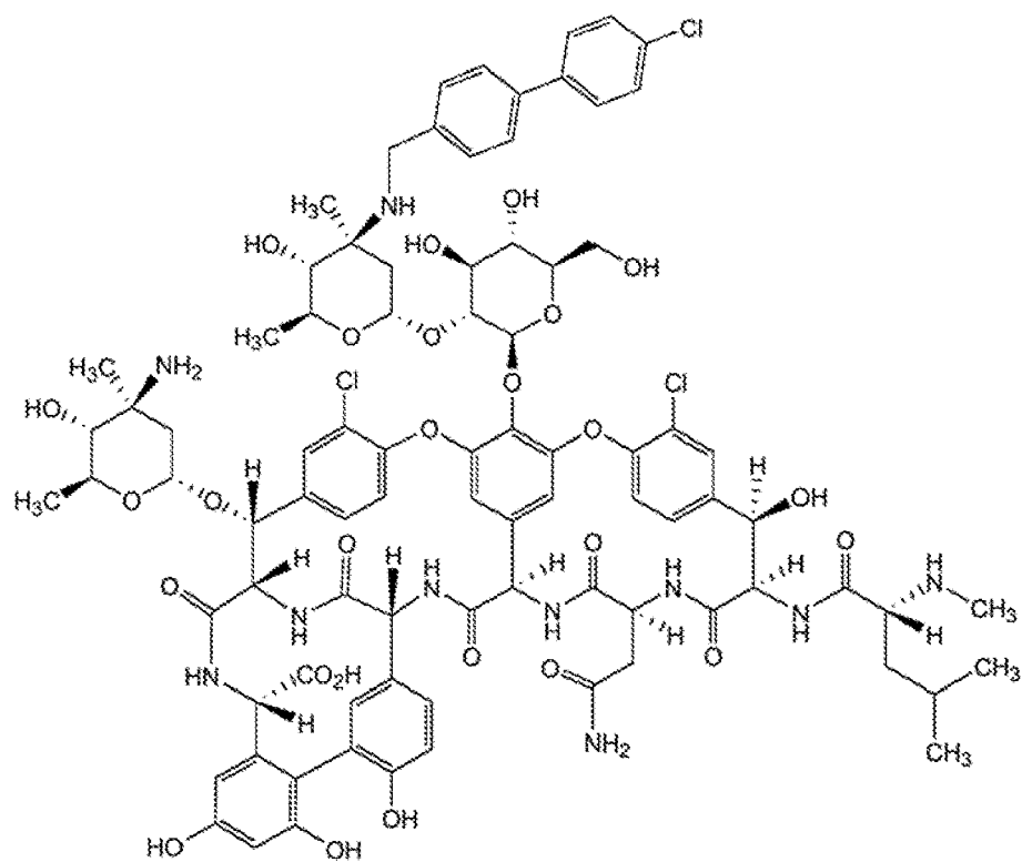
Oritavancin
