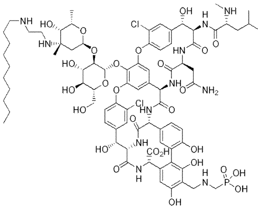
Telavancin
