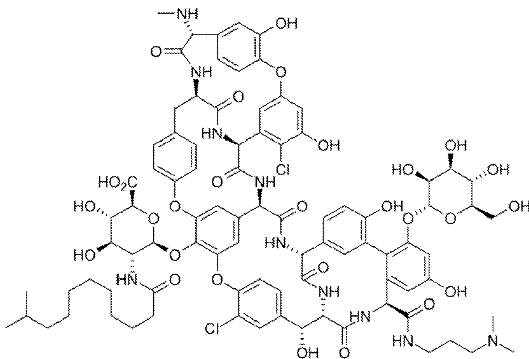
Dalbavancin
