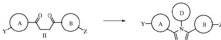
Scheme VI
