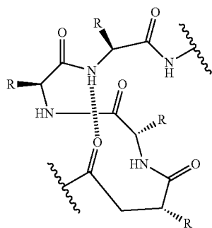
\alpha -helix
