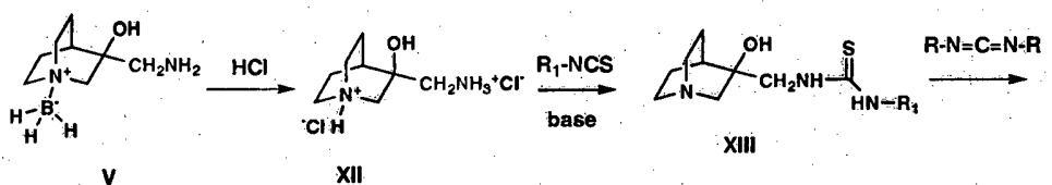
Scheme 2a.
