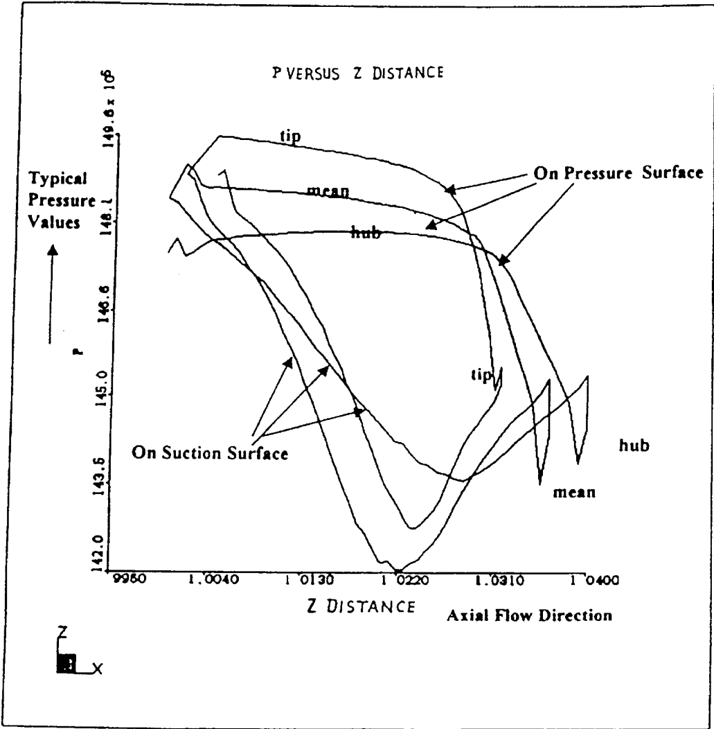
Fig. 12 : Surface Pressure Distribution : 3dsl_r Blade
