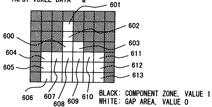
FIG. 34 A INPUT VOXEL DATA "a"
