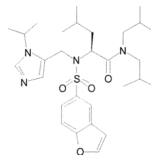
Cmpd. 142
