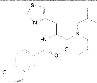
Cmpd. 55
