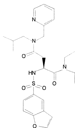
Cmpd. 39
