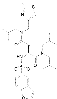
Cmpd. 129
