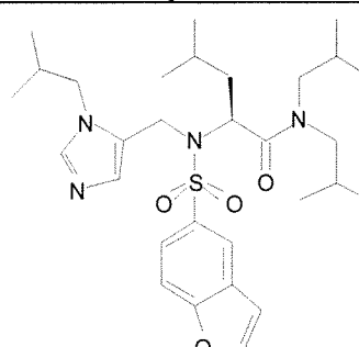
Cmpd. 146
