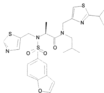
Cmpd. 158
