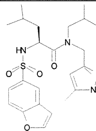
Cmpd. 30
