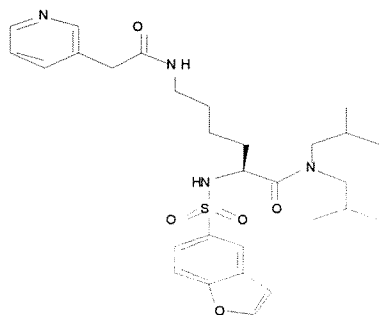
Cmpd. 33
