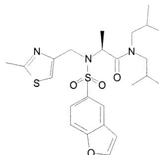
Cmpd. 168
