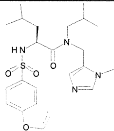
Cmpd. 29
