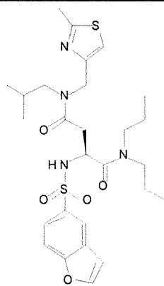
Cmpd. 143
