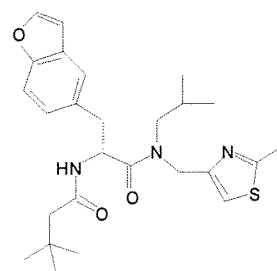
Cmpd. 162
