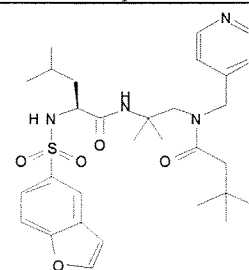
Cmpd. 28
