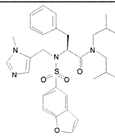
Cmpd. 124
