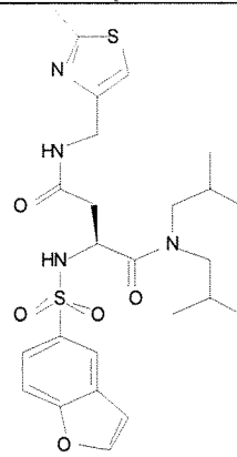
Cmpd. 46
