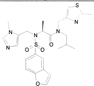
Cmpd. 163
