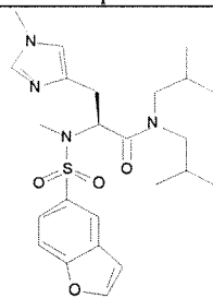
Cmpd. 51
