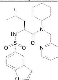
Cmpd. 24
