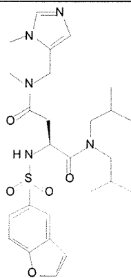
Cmpd. 139
