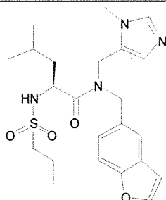
Cmpd. 149
