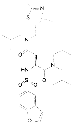
Cmpd. 127
