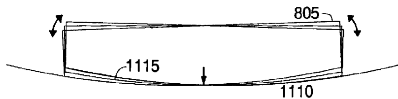
FIG. 35E
