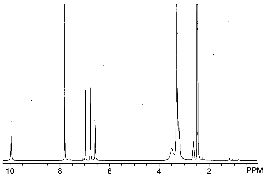
Proton NMR of Bis(triiodothyroninato)zinc
