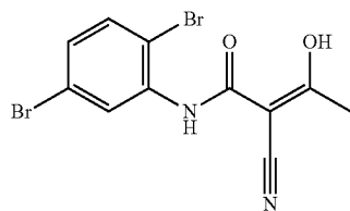
LFM-A13
