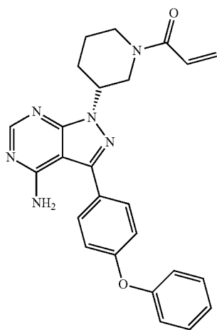
Ibrutinib
