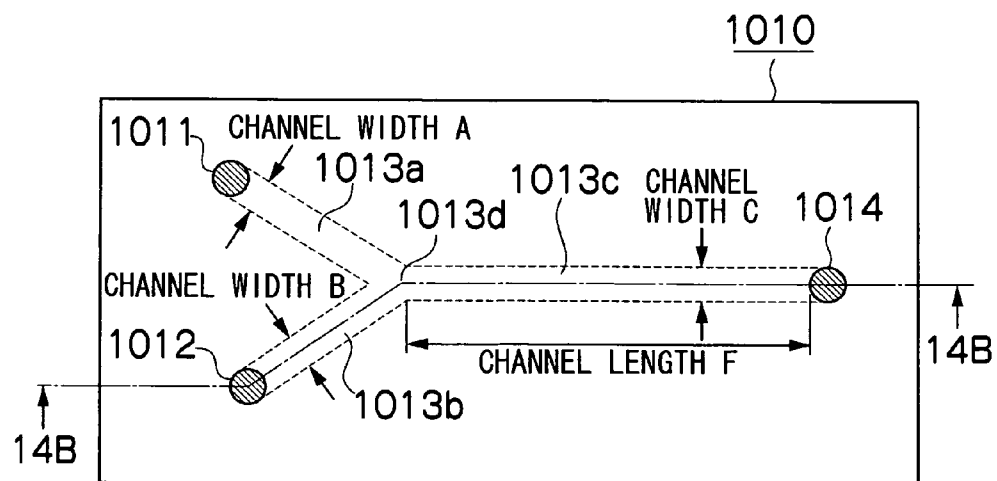
FIG.14A
