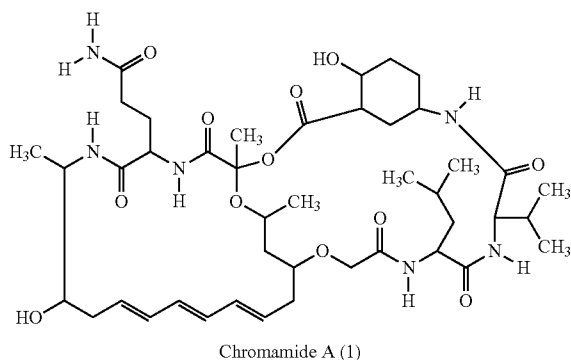
Chromamide A (1)
