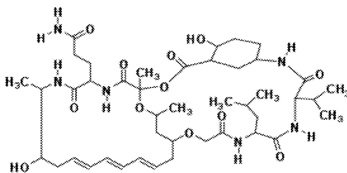
Chromamide A (1)
