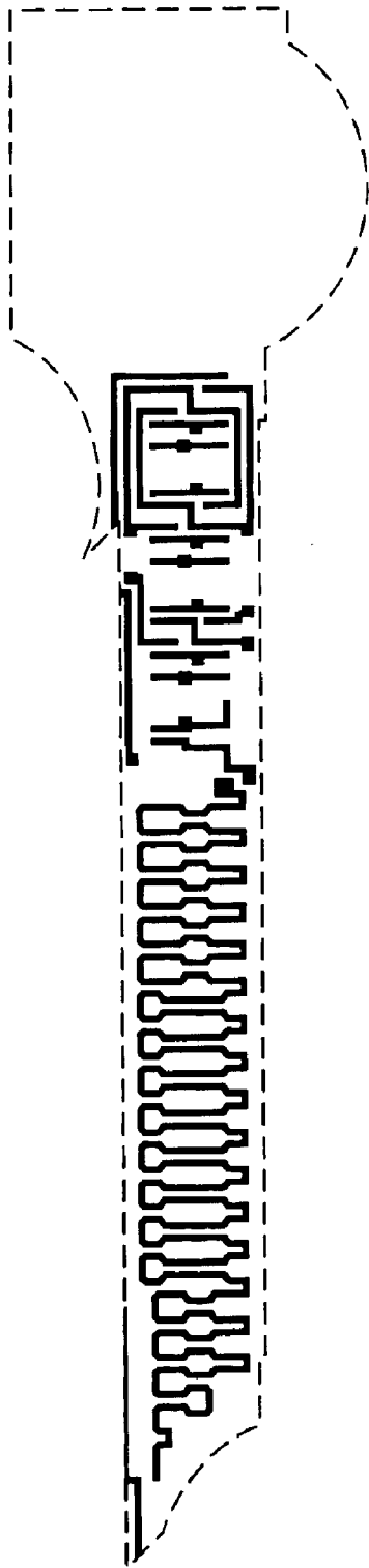
Poly mask
