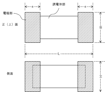
チップコンデンサ (10 pF ~ 47 \mu F) サイズ表
