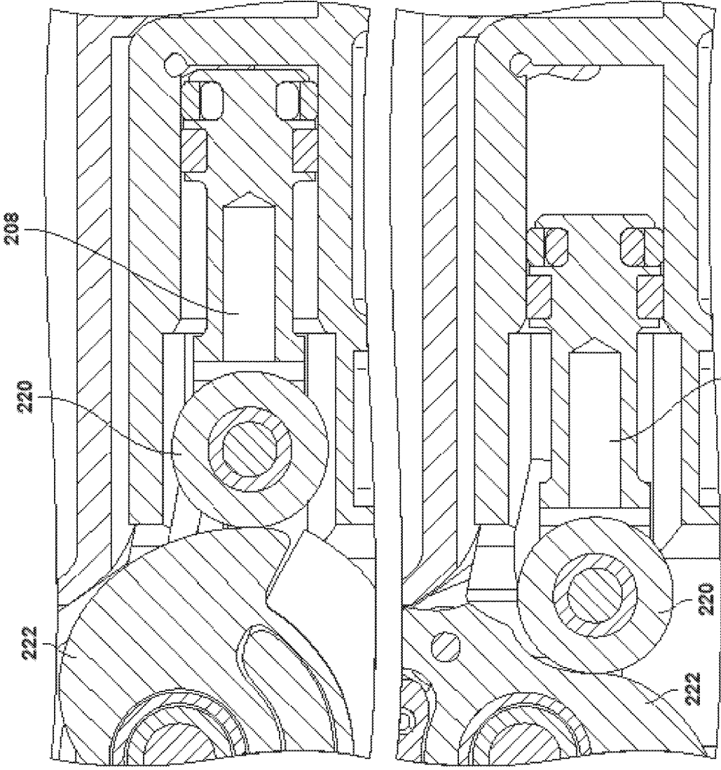
FIG. 2E
