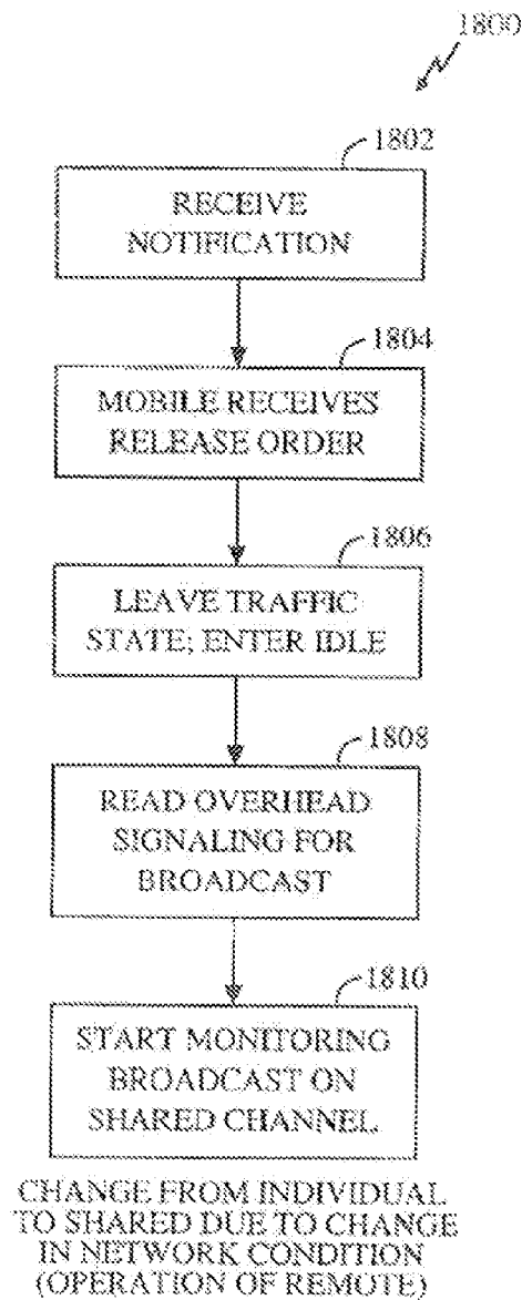
FIG. 18
