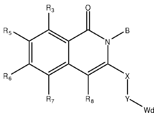
Formula IC
