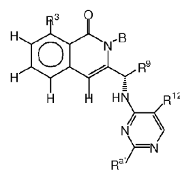
Formula XIV-A2
