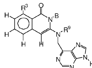
Formula VI-A
