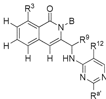
Formula (XIV-A).
