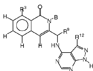
Formula XI-A
