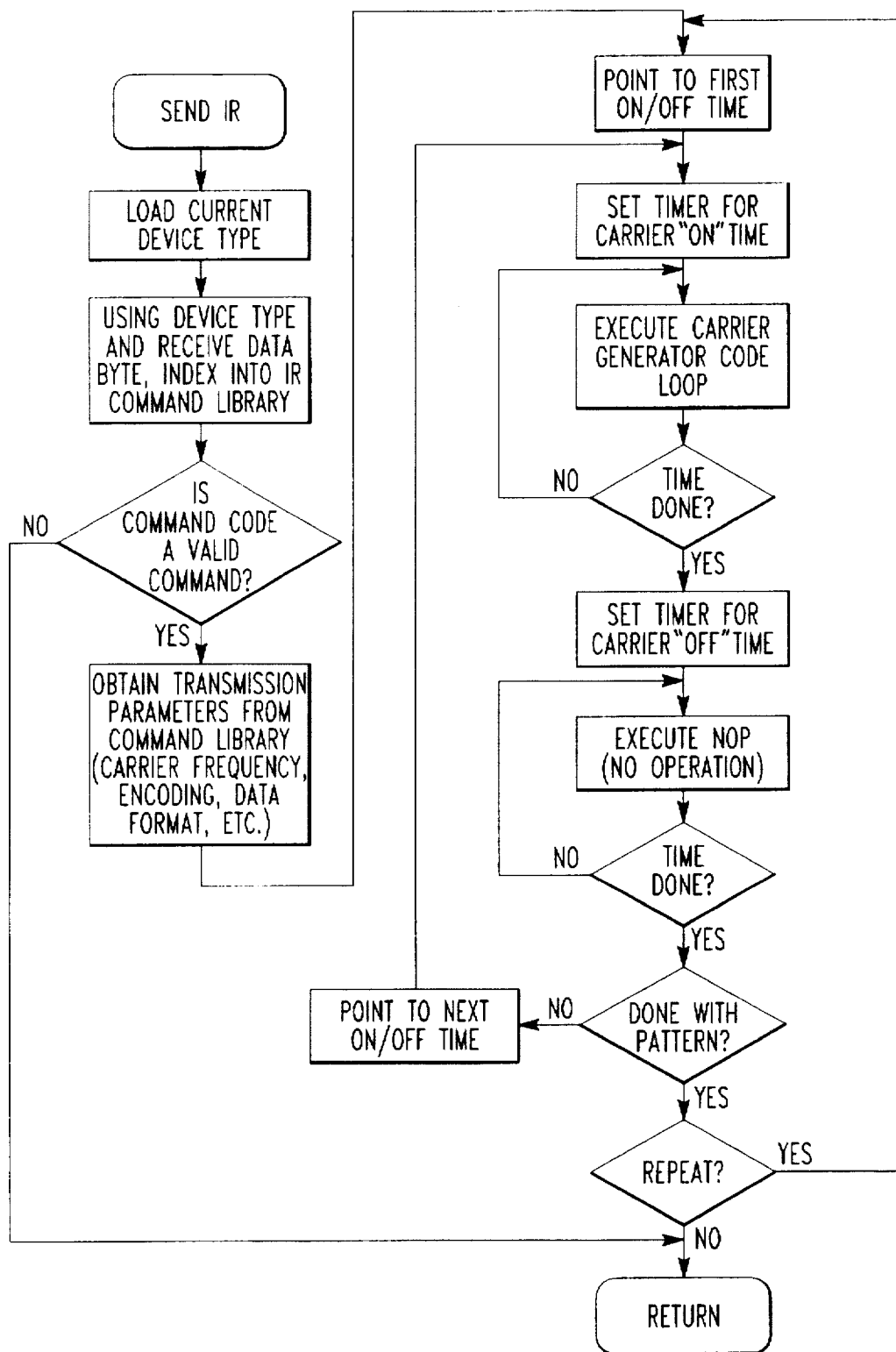
FIG. 6 SEND IR COMMAND
