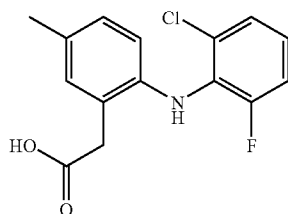
Lumiracoxib
